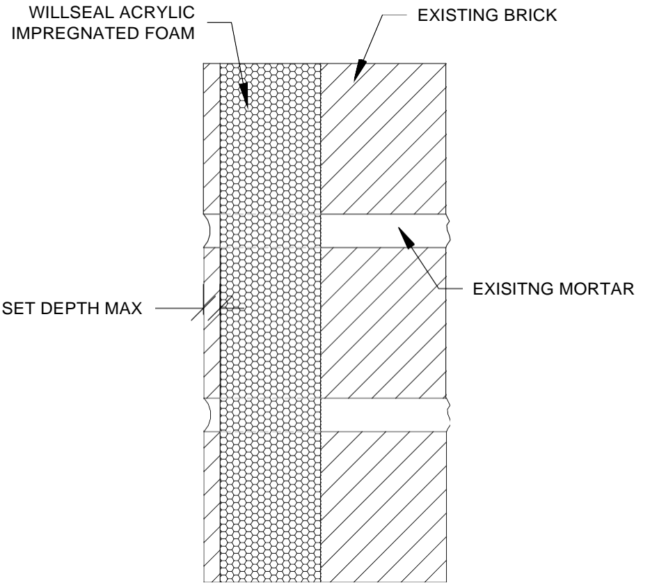
1 SECTION VIEW N.T.S.
