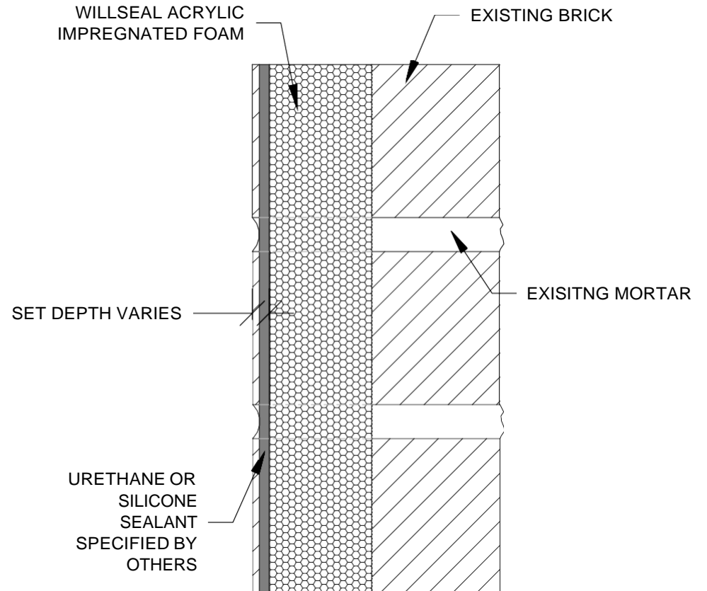
1 SECTION VIEW N.T.S.
