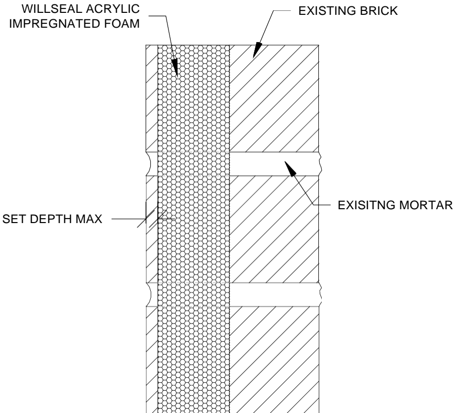
1 SECTION VIEW N.T.S.
